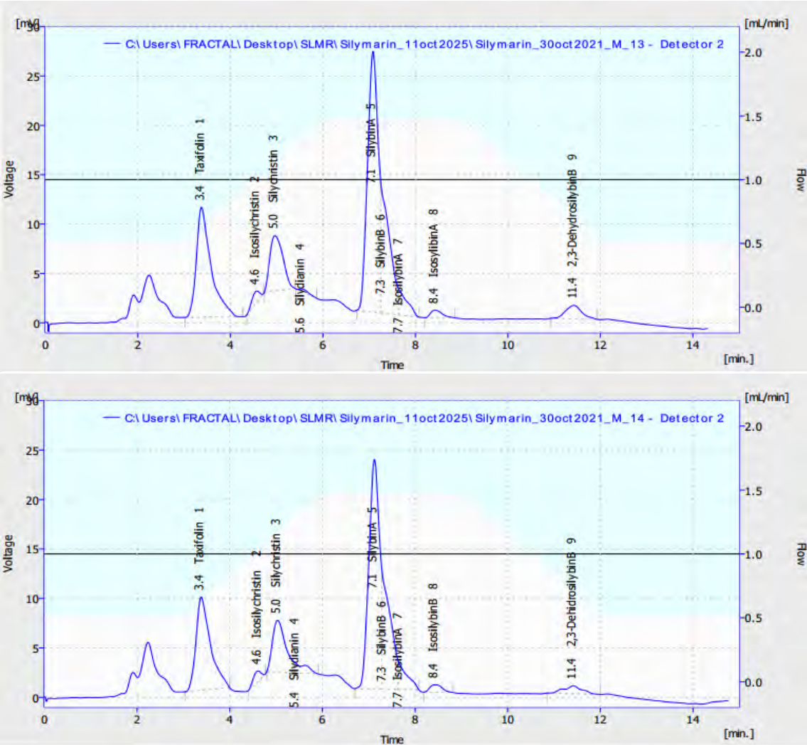
Figura 49 Cromatogramas HPLC-DAD de flavonolignanos de silimarina en semillas fértiles e infértiles procedente de la Comunidad Fortaleza Sacsayhuaman
