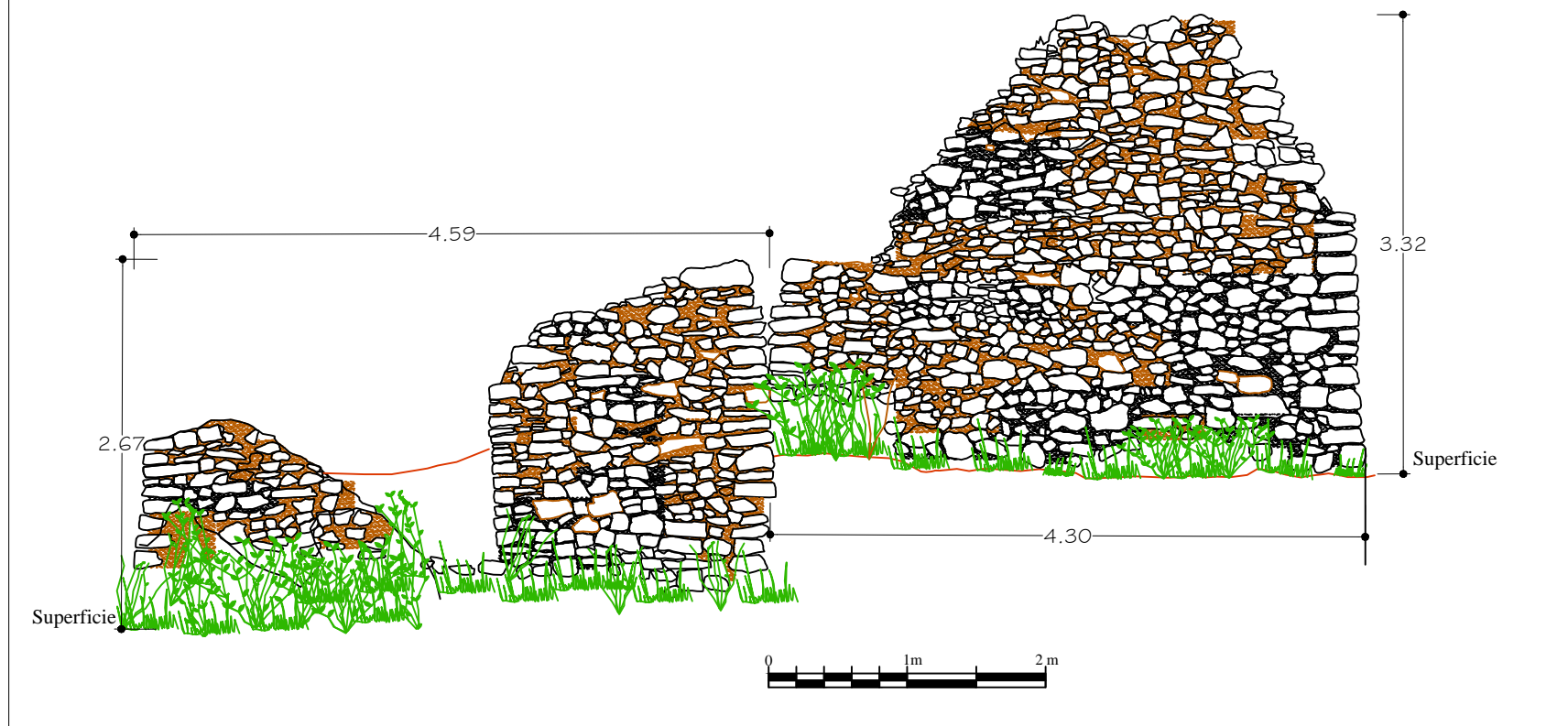
Elevación del lado exterior del R-4
